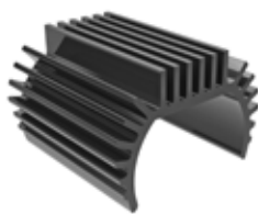
Art.Nr.: TRX9793-GRAY TRAXXAS TRX-4M Kühlkörper 6061-T6 Alu dunkelgrau eloxiert
